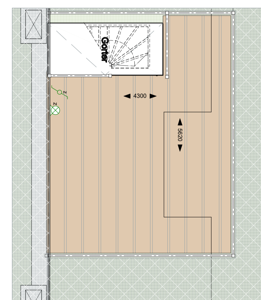
Dakterras - 1:50
