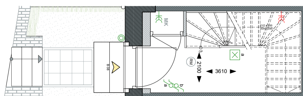
Begane grond - 1:50
